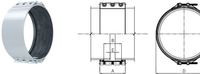
E = Espace maximum entre les deux tubes = 15 mm A = Largeur = 200 mm
