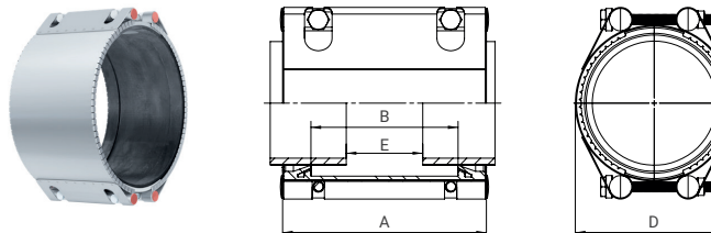
E = Espace maximum entre les deux tubes = 15 mm A = Largeur = 200 mm
