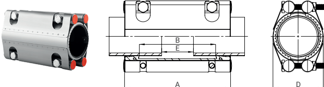
E = Espace maximum entre les deux tubes = 15 mm A = Largeur = 200 mm
