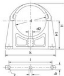
Diamètres 40 à 160 mm
